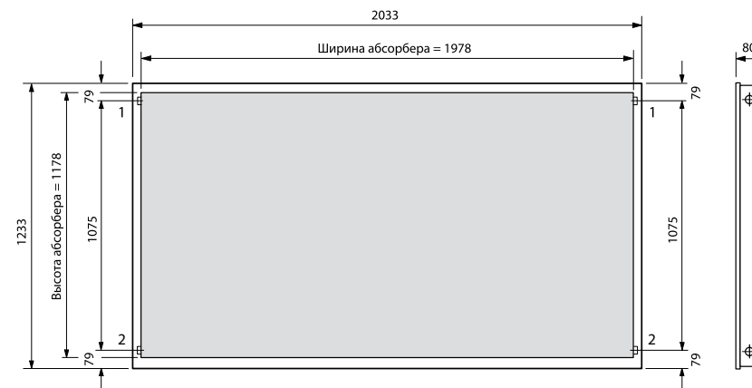
auroTHERM VFK 145 H
