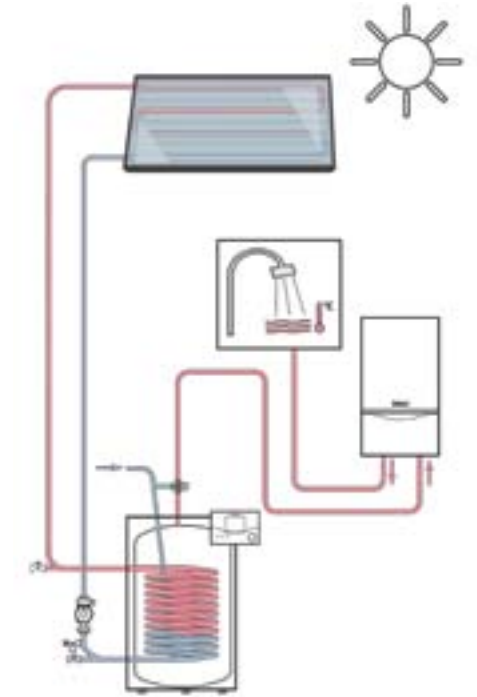
Солнечная установка auroSTEP plus 1.150 HT
